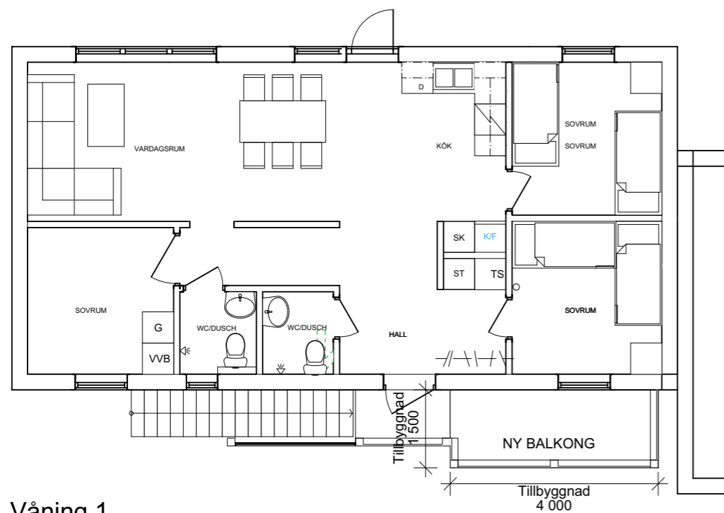
Våning 1 1:100
