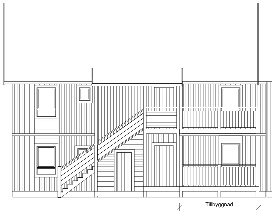
Fasad entrésidan 1:100
