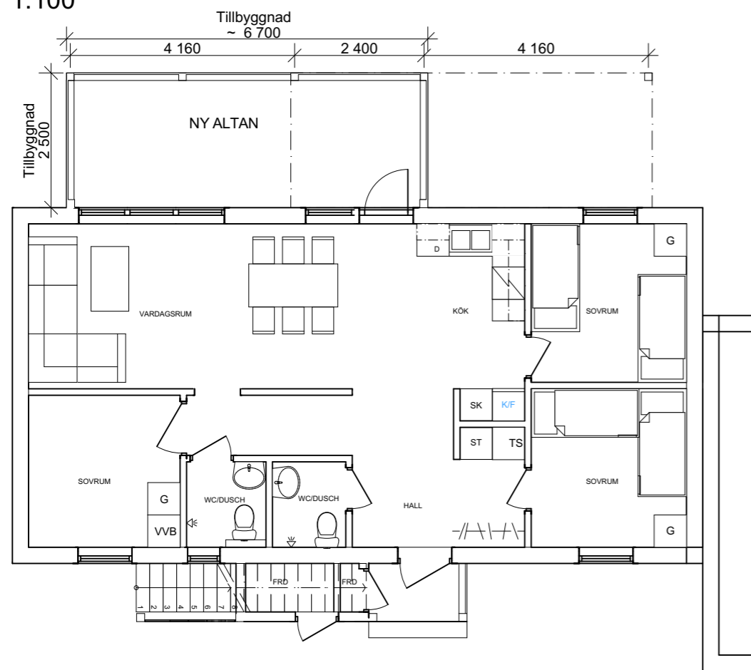
Våning 1 1:100
