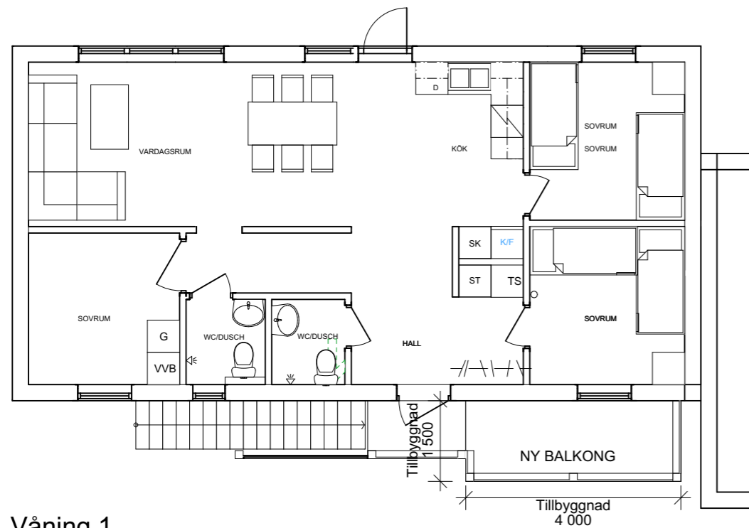
Våning 1 1:100
